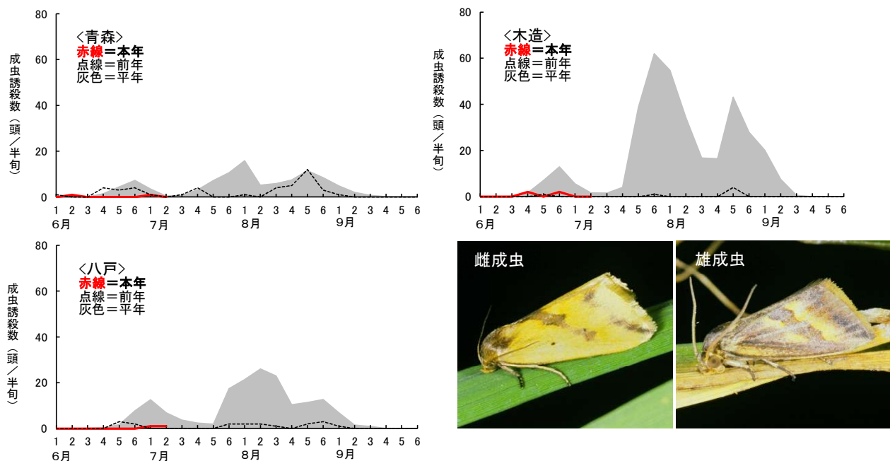
図5 予察灯によるフタオビコヤガの半旬別誘殺数 ※木造において、7月2半旬の値は欠測値（7月7～10日）を含む。
